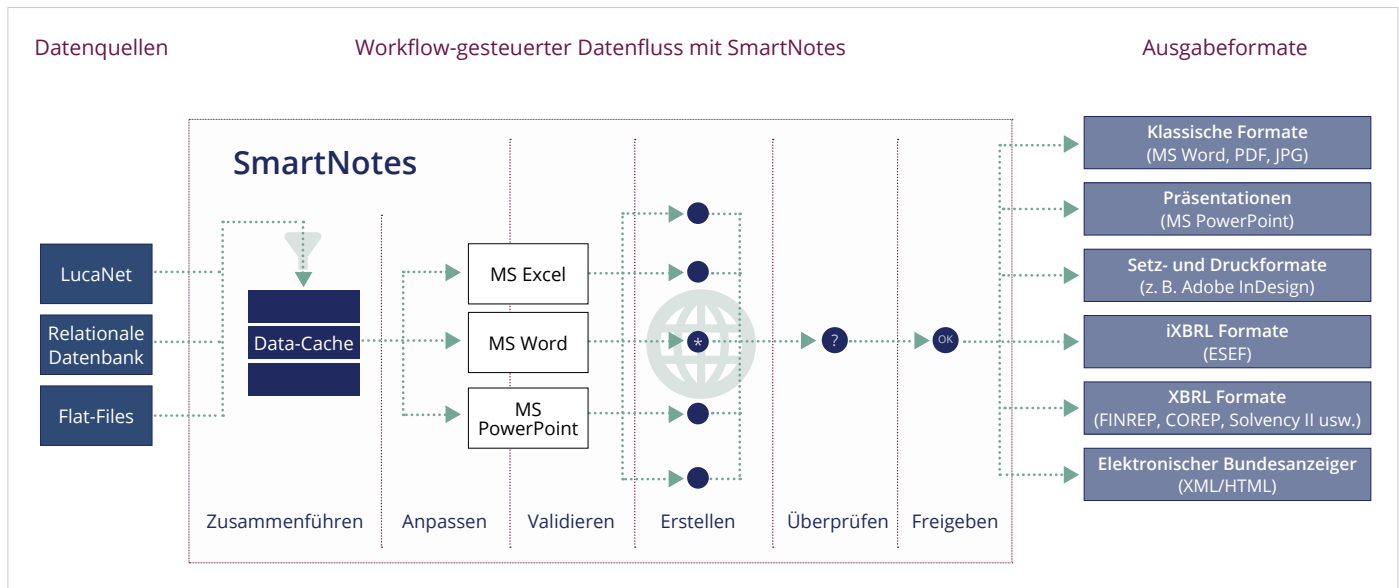
Abbildung 2: Geschäftsbericht-Workflow mit SmartNotes
